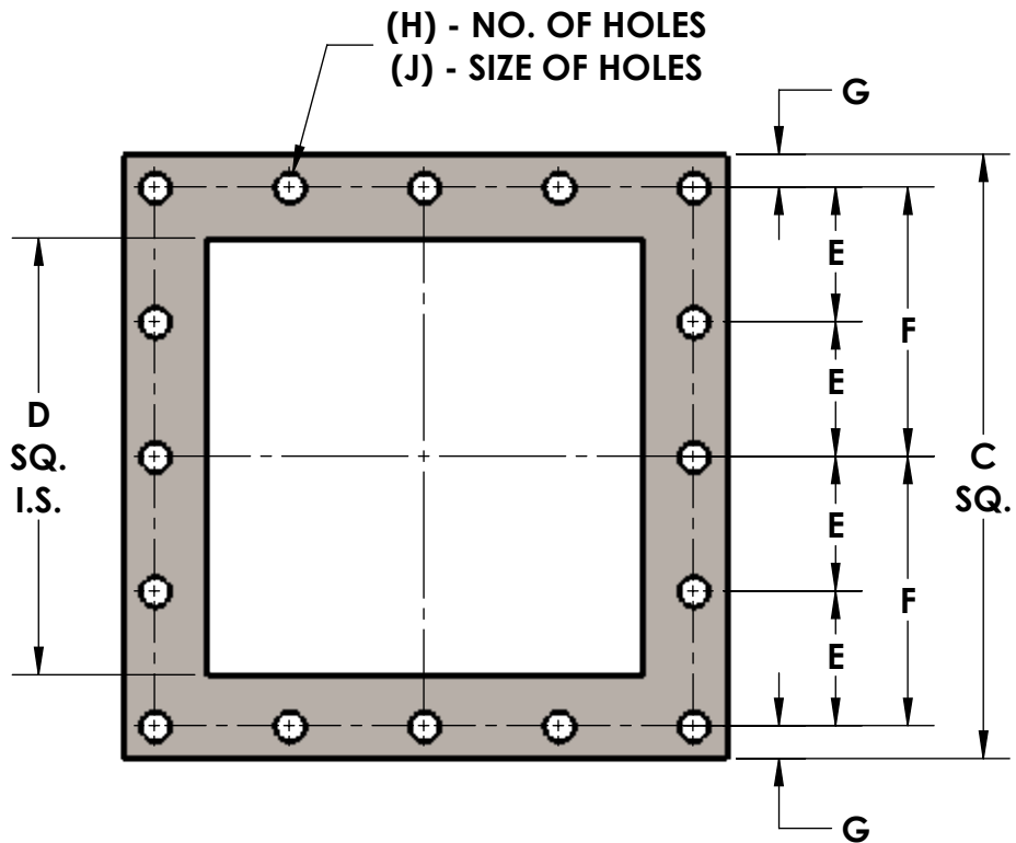
DETAIL: DISCHARGE FLANGE
